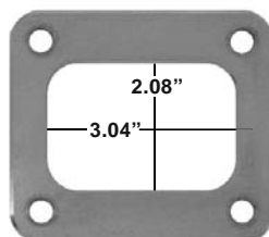
3.00" Rectangle
